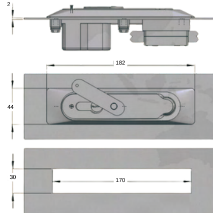
ZINC DIE-CAST CYLINDER 1810-HT-8.1
